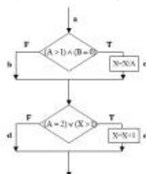
图 1 语句覆盖的例子
